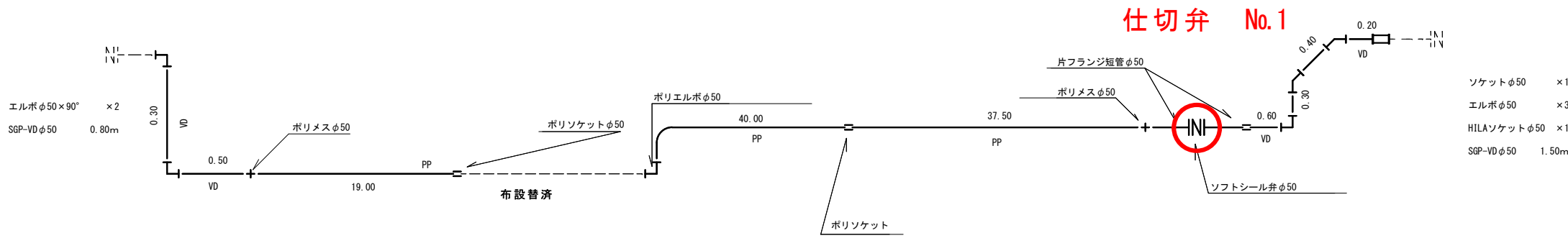
3工区 配管図 S=free
