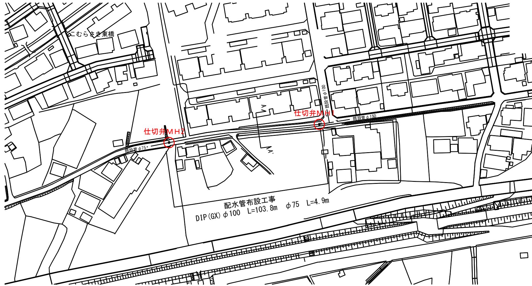
平面図 S=1/2000
