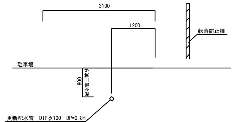
横断面図A-A' S=1:60
