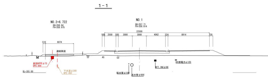
横断面図 S=1:200
